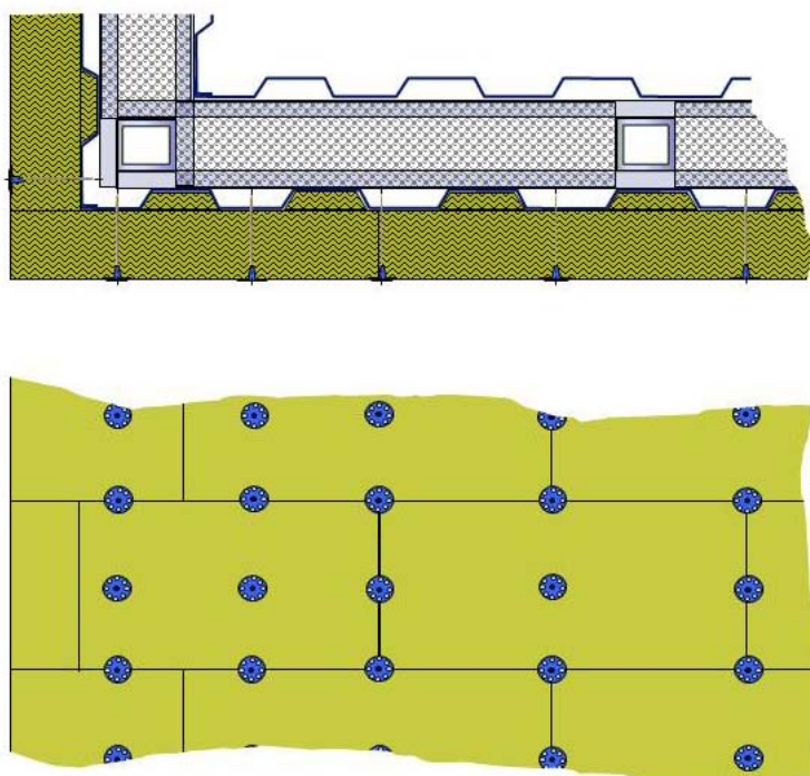
Obr. 5b - Kladení fasádních tepelně izolačních desek na plechový podklad (nesmí vzniknout průběžná vertikální mezera větší jak 0,01 m 2 )
