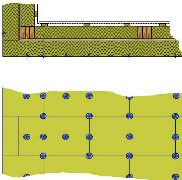
Obr. 5a - Kladení fasádních tepelně izolačních desek na deskový podklad
