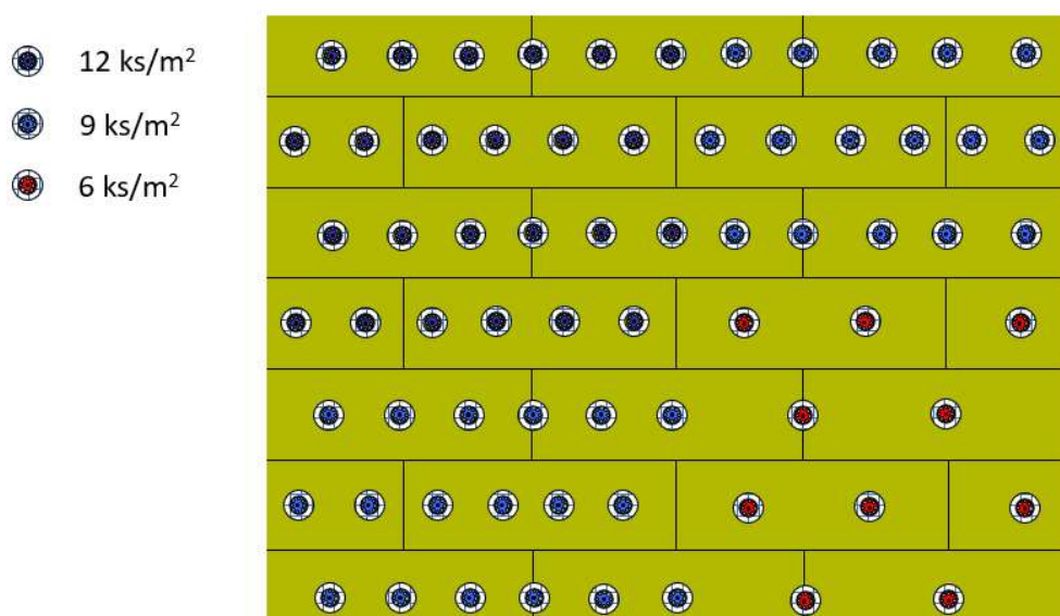
Obr. 6b Příklady rozmístění kotvicích hmoždinek příčné vlákno 333 x 1000; TR80 schéma kotvení
