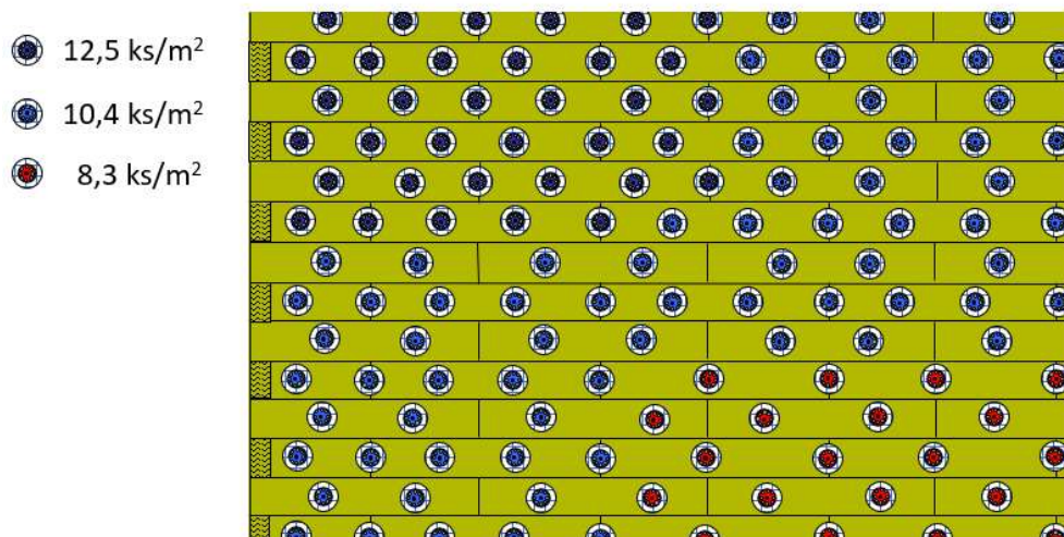
Obr. 6b Příklady rozmístění kotvicích hmoždinek příčné vlákno 333 x 1000; TR80 schéma kotvení
