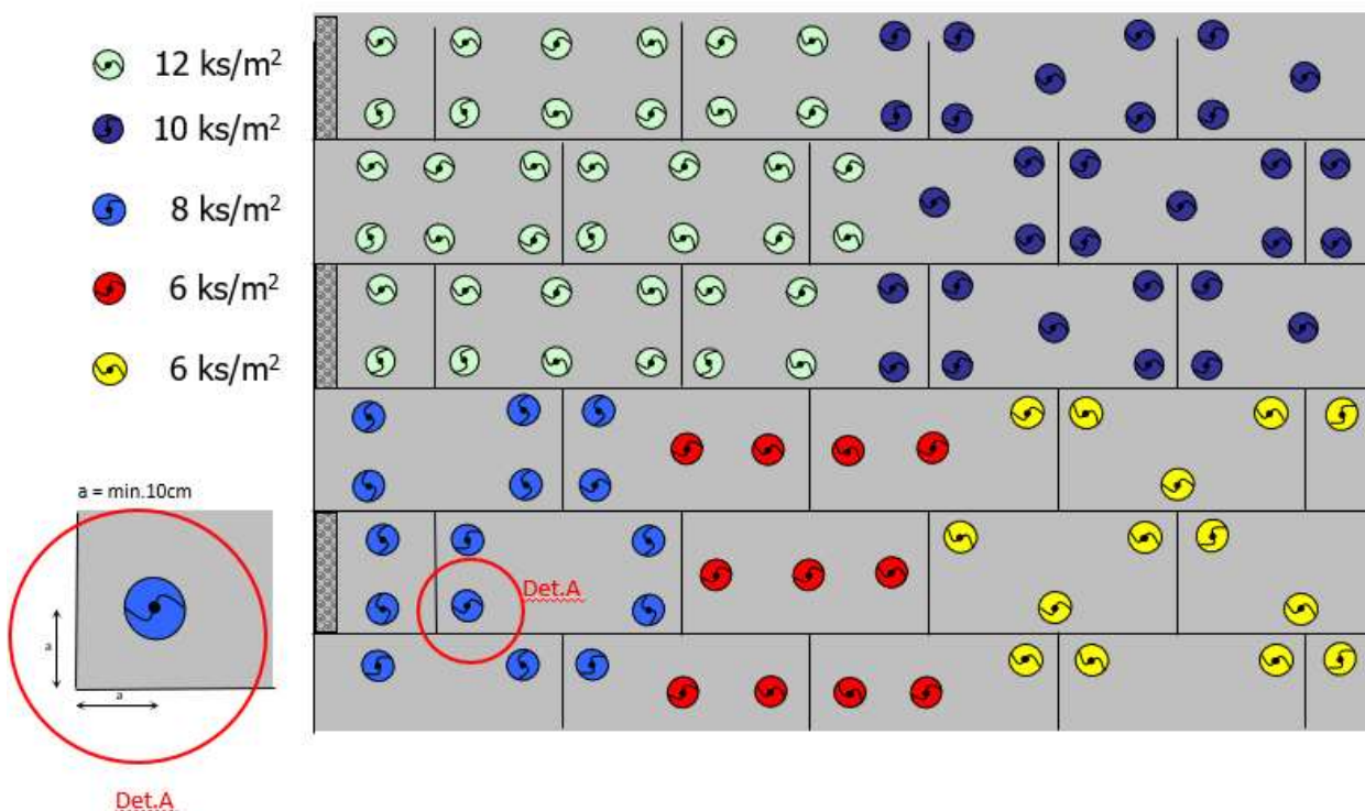
Obr. 6b Příklady rozmístění kotvicích hmoždinek fischer Termoz ecotwist II SV
