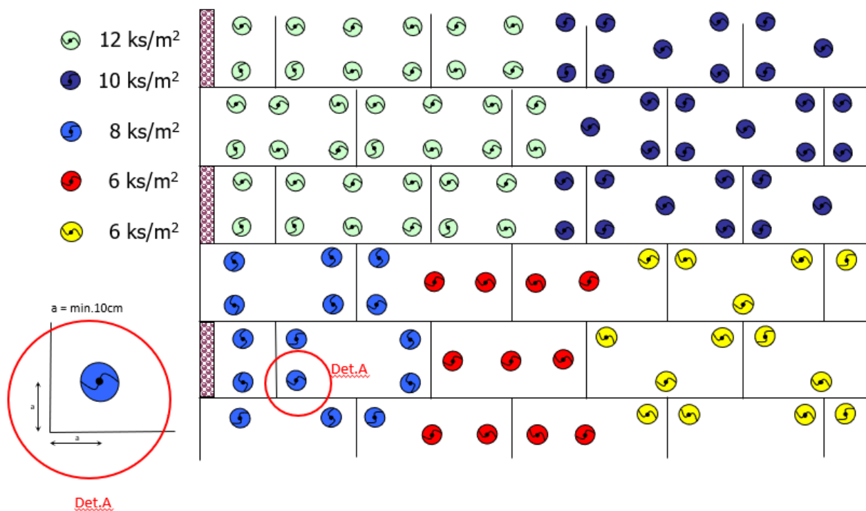
Obr. 6b Příklady rozmístění kotvicích hmoždinek fischer Termoz ecotwist II SV
