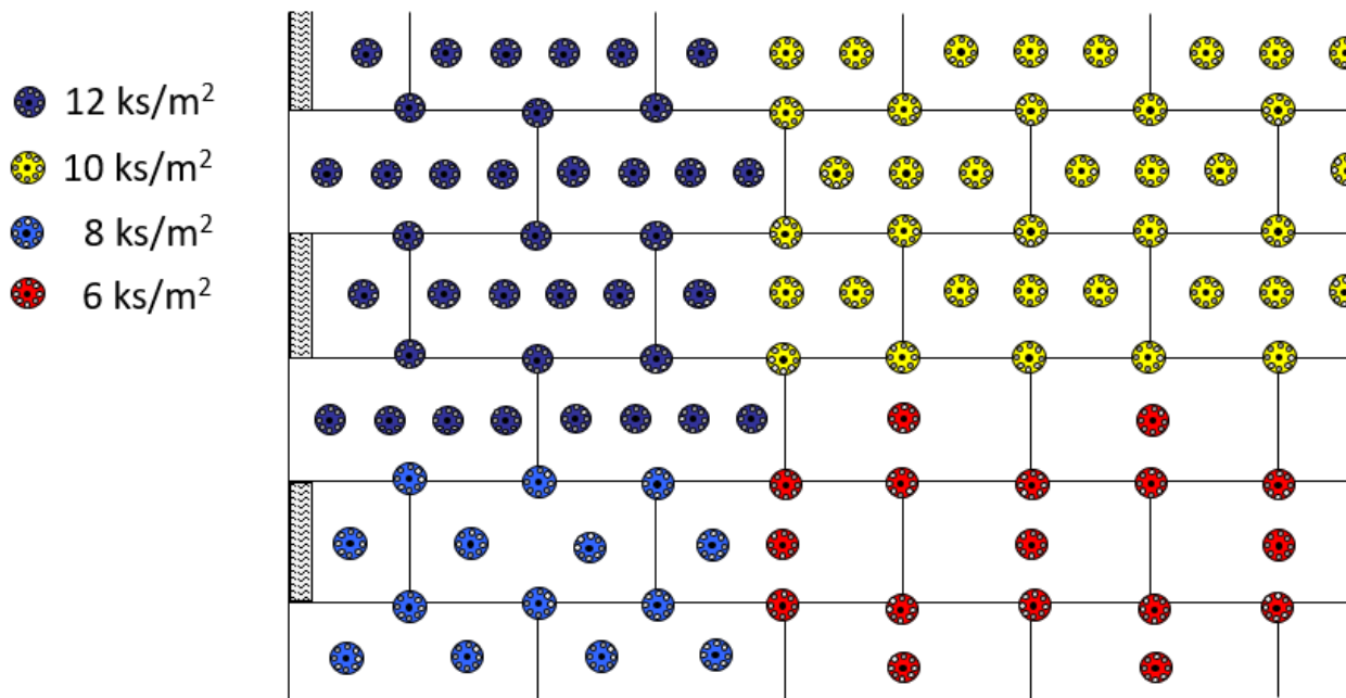
Obr. 6b Příklady rozmístění kotvicích hmoždinek fischer Termoz ecotwist II SV
