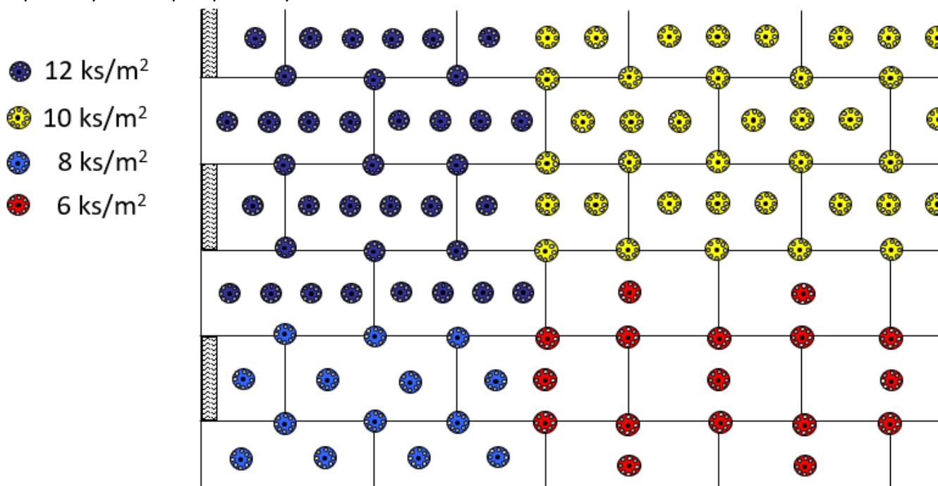
Obr. 6 Příklady rozmístění kotvicích prvků Doporučený kotevní plán pro desky 500x1000
