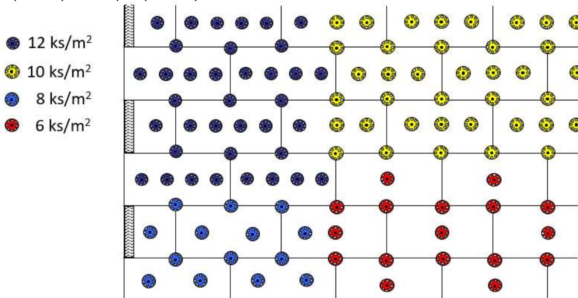
Obr. 6a Příklady rozmístění kotvicích hmoždinek
