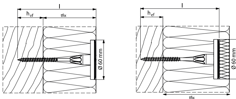
Povrchová montáž
